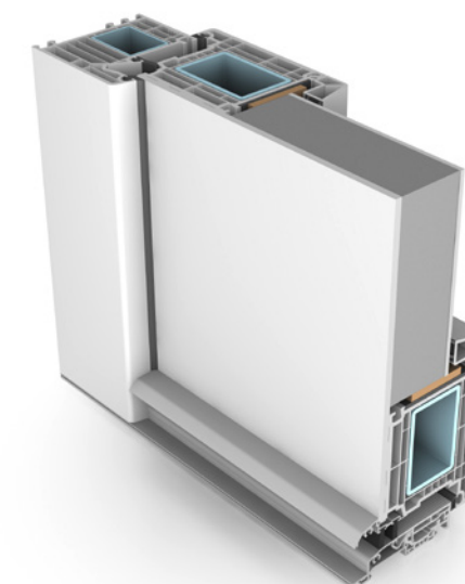
Für Haustüren mit flügelüberdeckenden Füllungen und einer durchgängigen Außenfläche ohne störende Schattenfugen bietet das System SOFTLINE 82 ein speziell entwickeltes Flügelprofil
